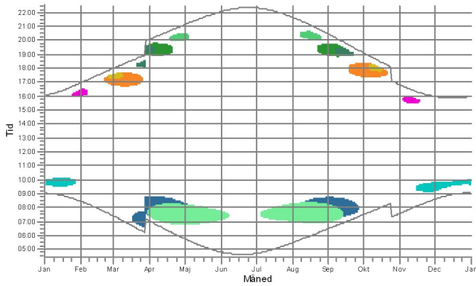
9: VESTAS V117-3.3 MW 3300 117.0 !O! nav: 91,5 m (TOT:150,0 m) (2)
